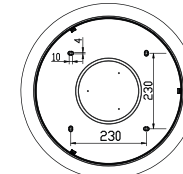
Отверстия для монтажа SATURN RGB 60W R
