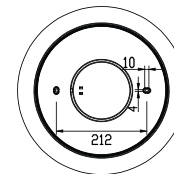
Отверстия для монтажа SATURN RGB 25W R
