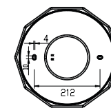
Отверстия для монтажа ALMAZ RGB 25W R
