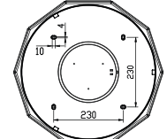
Отверстия для монтажа ALMAZ RGB 60W R
