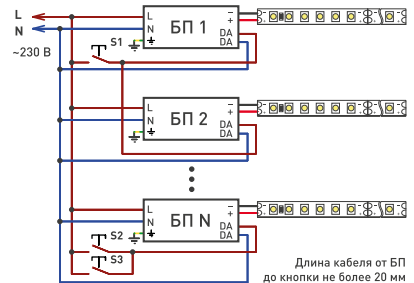
Рис.3. Структурная схема соединения оборудования при использовании управления PUSH DIM
