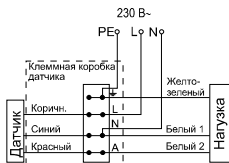
Рисунок 18 – Схема подключения датчиков ДД-017, ДД-019
