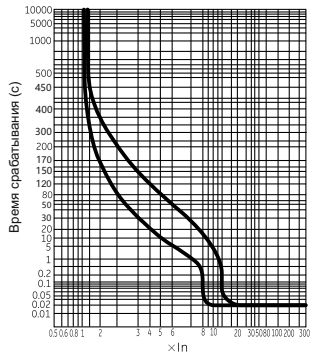
г) Времятоковые характеристики выключателей BA88-37
