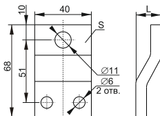
г) Наконечник-переходник для ВА88-40
