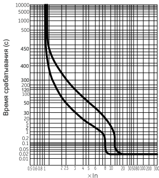
в) Времятоковые характеристики выключателей BA88-35
