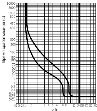
д) Времятоковые характеристики выключателей ВА88-40
