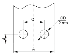
б) Шина для ВА88-40
