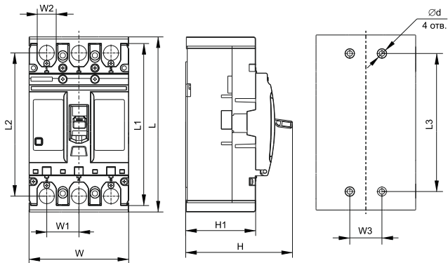
Рисунок 4 – Габаритные и установочные размеры выключателей
