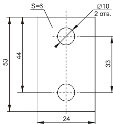
в) Наконечник-переходник для ВА88-37
