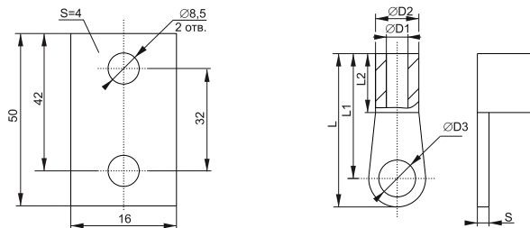
а) Наконечник-переходник для ВА88-32
