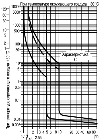
Рисунок 1 – Характеристика C
